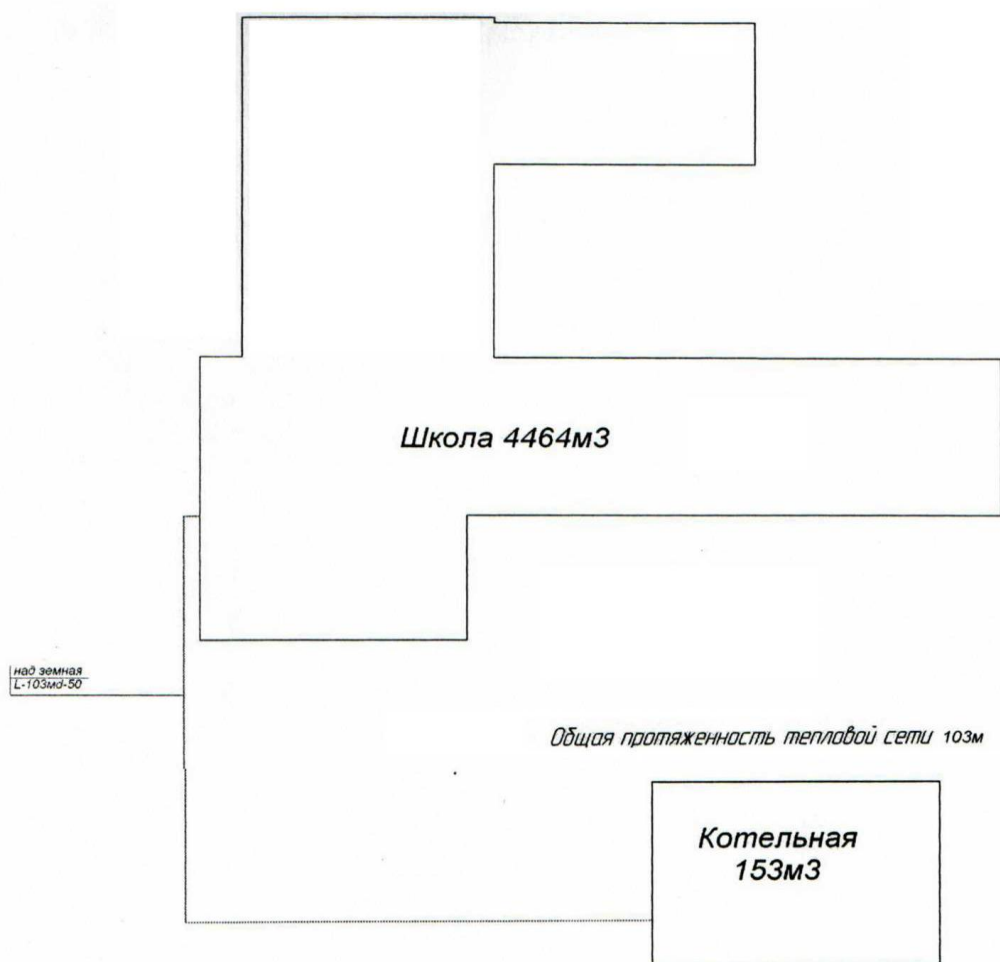
Рис. 4. Схема тепловых сетей котельной №5 д. Усть-Тарсьма, ул. Школьная Титовского сельского поселения
