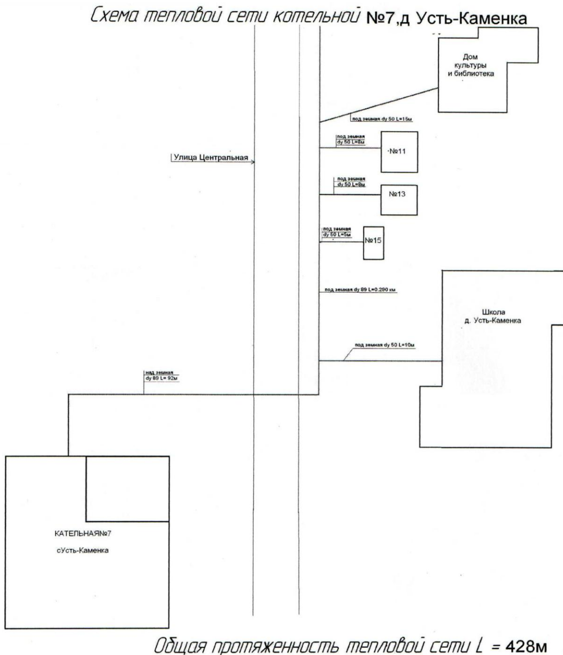
Рис. 5. Схема тепловых сетей котельной №7 д. Усть-Каменка, ул. Центральная Титовского сельского поселения
