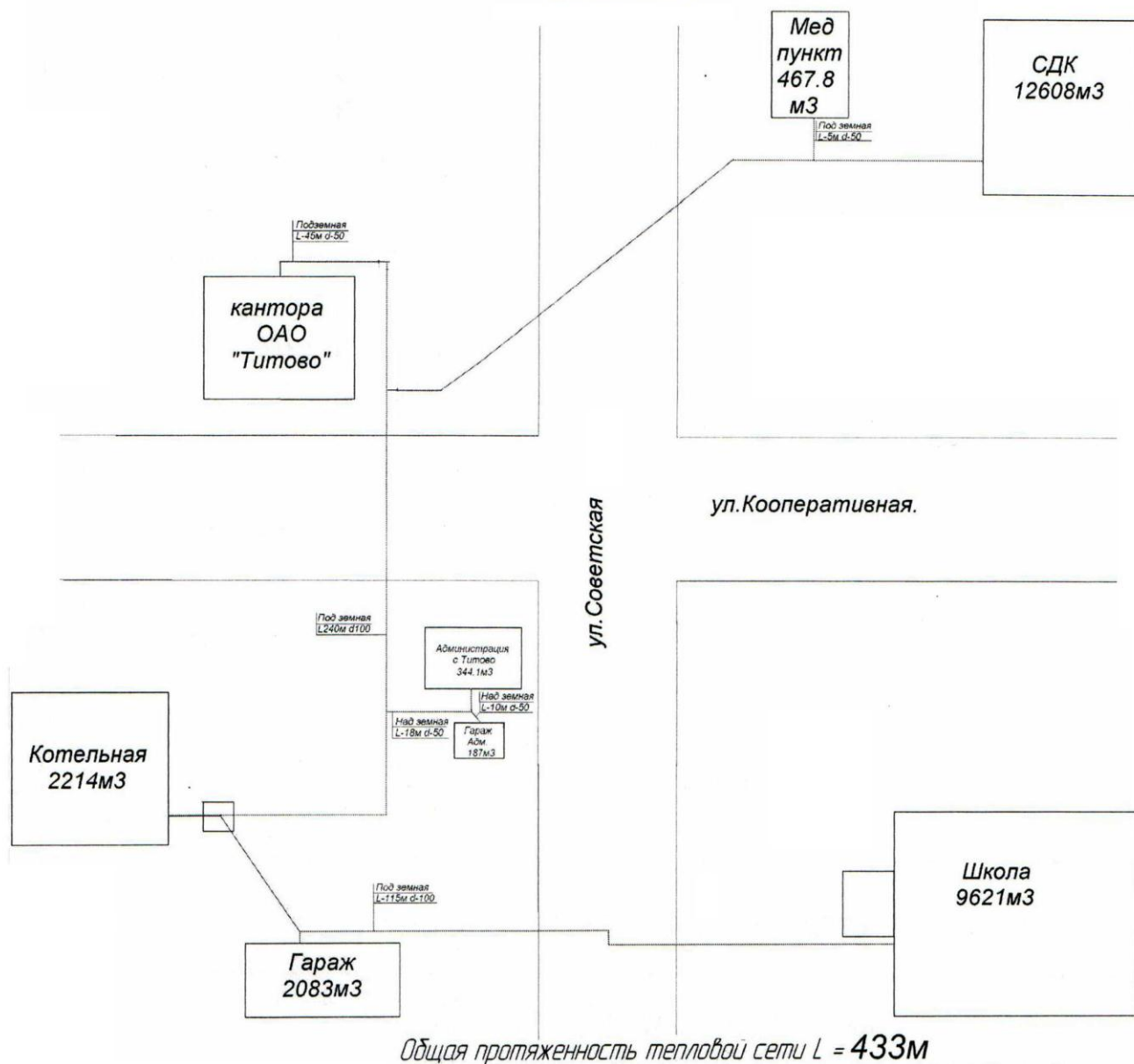
Рис. 6. Схема тепловых сетей котельной №6 с. Титово, ул. Советская Титовского сельского поселения
