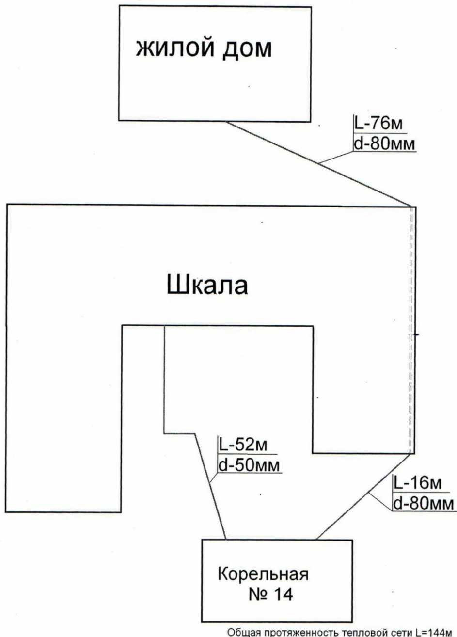
Рис. 7. Схема тепловых сетей котельной № 14 д. Шури́нка, пер. Школьный Тарасовского сельского поселения
