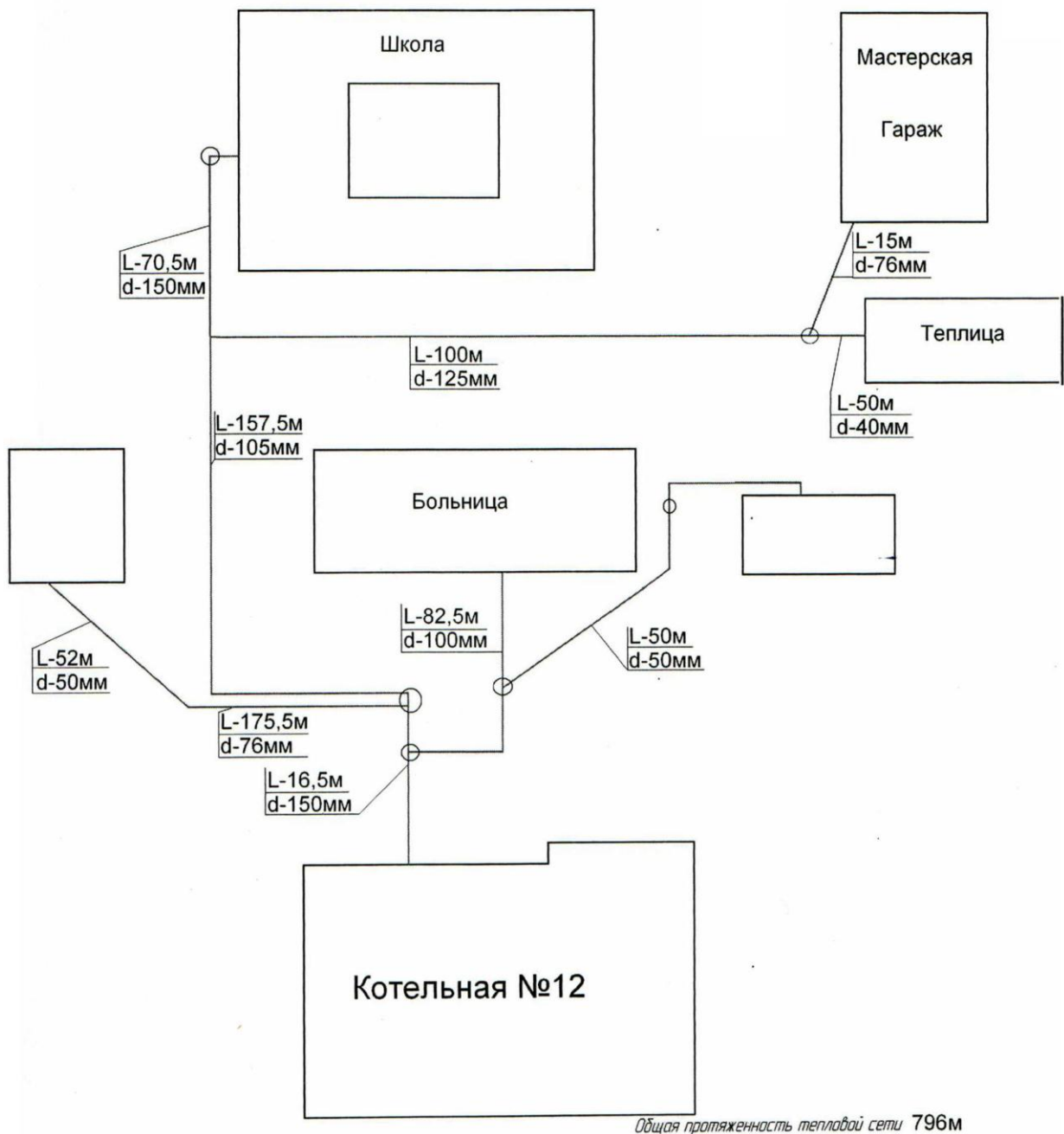
Рис. 5. Схема тепловых сетей котельной № 12 с. Тарасово, ул. Центральная 96 Тарасовского сельского поселения
