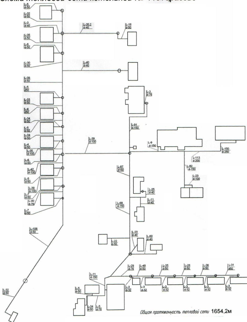
Схема тепловой сети котельной № 11 с.Тарасово
